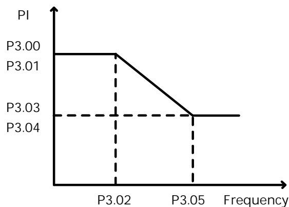
Graph 4-5 PI parameters
